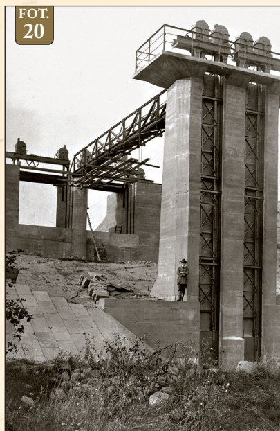
Fot. 20 – Wieża zasuw upustu głębinowego zapory, obecnie pod wodą, listopad 1920 roku
